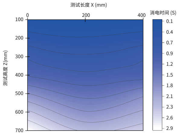
500mm 棒长 AP-AB1228 在 0.3MPa 气流压力下的放电时间分布图
