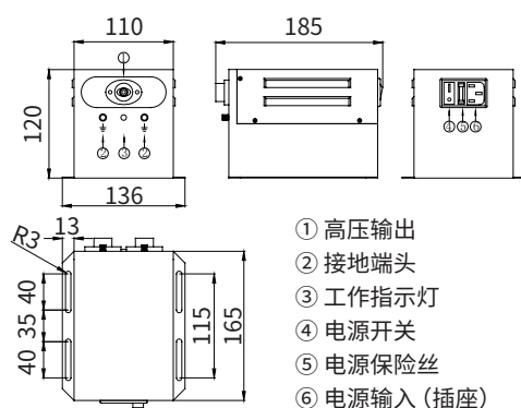
AP-AY1504 结构尺寸图
