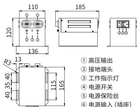
AP-AY2504 结构尺寸图
