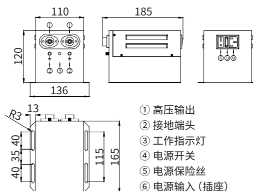
AP-AY2506 结构尺寸图
