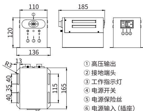
AP-AY1506 结构尺寸图
