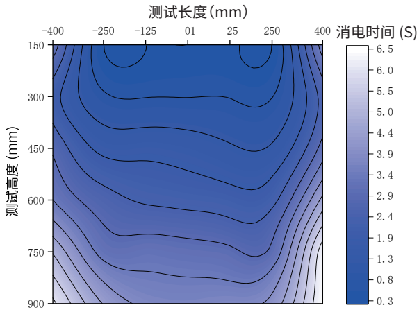
AP-DJ2813 消电时间空间分布图
