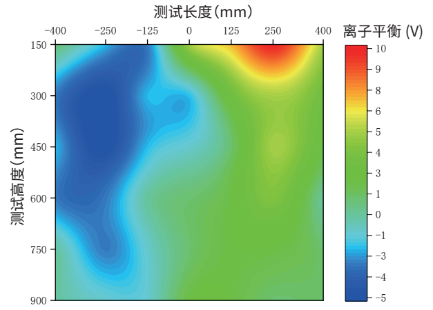
AP-DJ2813 离子平衡空间分布图
