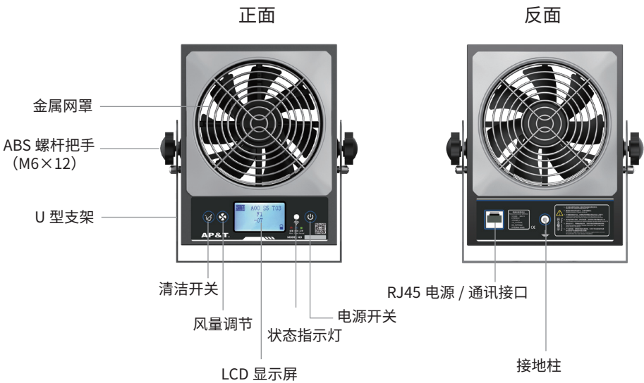
液晶屏参数显示说明
