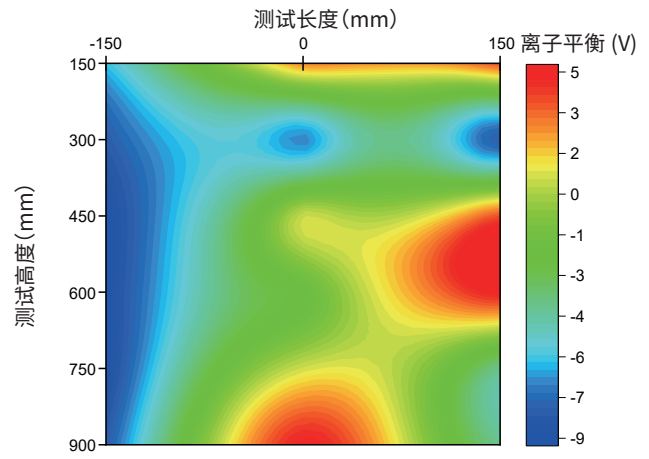
AP-DJ2811 离子平衡空间分布图
