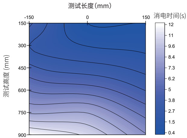
AP-DJ2811 消电时间空间分布图
