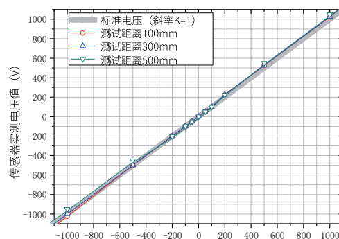
图 1-2 标准平板电极垂直测试数据图
