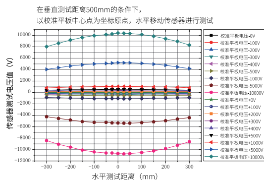
图 2-1 垂直距离 500mm 时，标准平板电极水平测试数据图
