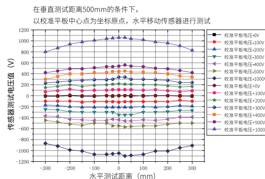
图 2-2 垂直距离 500mm 时，标准平板电极水平测试数据图
