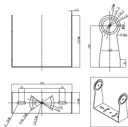
固定支架孔位图
