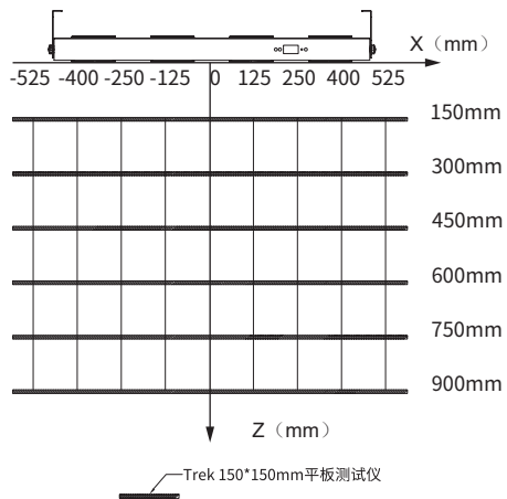
风机测试方位图
