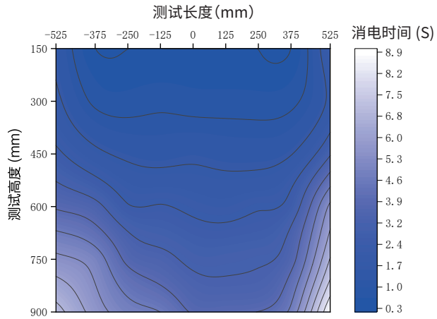
AP-DJ2814 消电时间空间分布图
